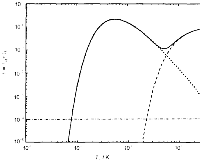
图 1 裸奇异星表面的电磁辐射流 [17]
